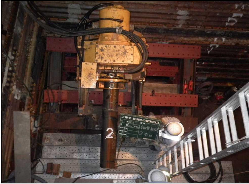
鋼管据付状況
